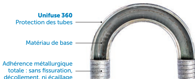
Vue en coupe d'un tube cintré
