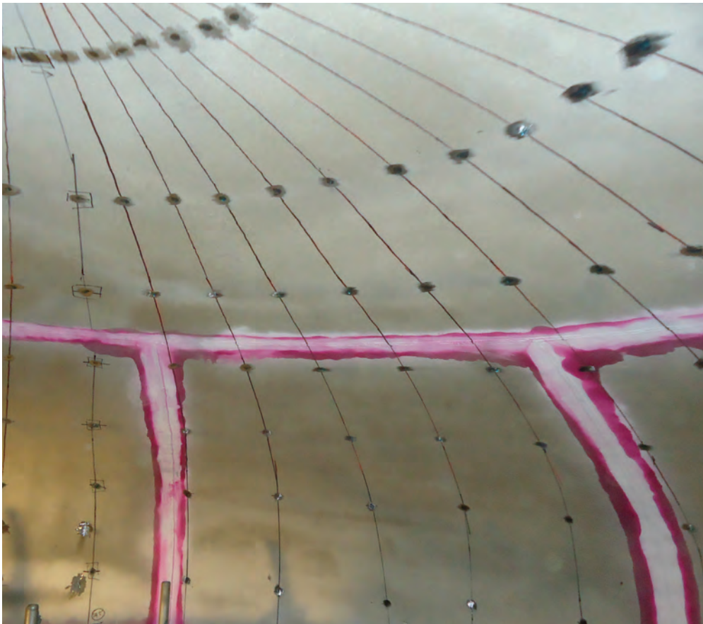
Controlli non distruttivi con liquidi penetranti
