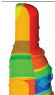
Simulazione a colori delle deformazioni in una Vacuum Tower
