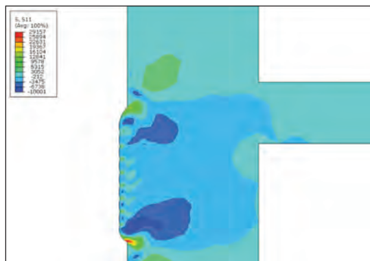
Previsione degli stress residui
