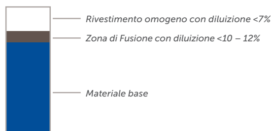
Illustrazione schematica di una sezione trasversale
